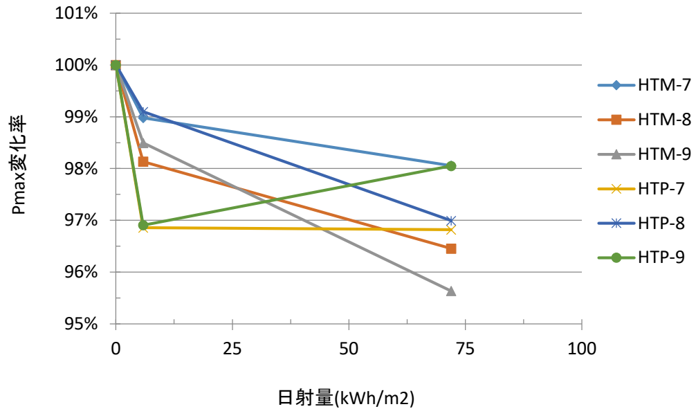
屋外暴露試験_中間結果
